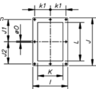
Bouche d'impulsion
