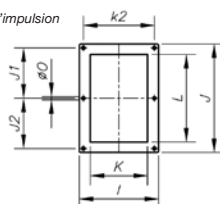
Bouche d'impulsion
